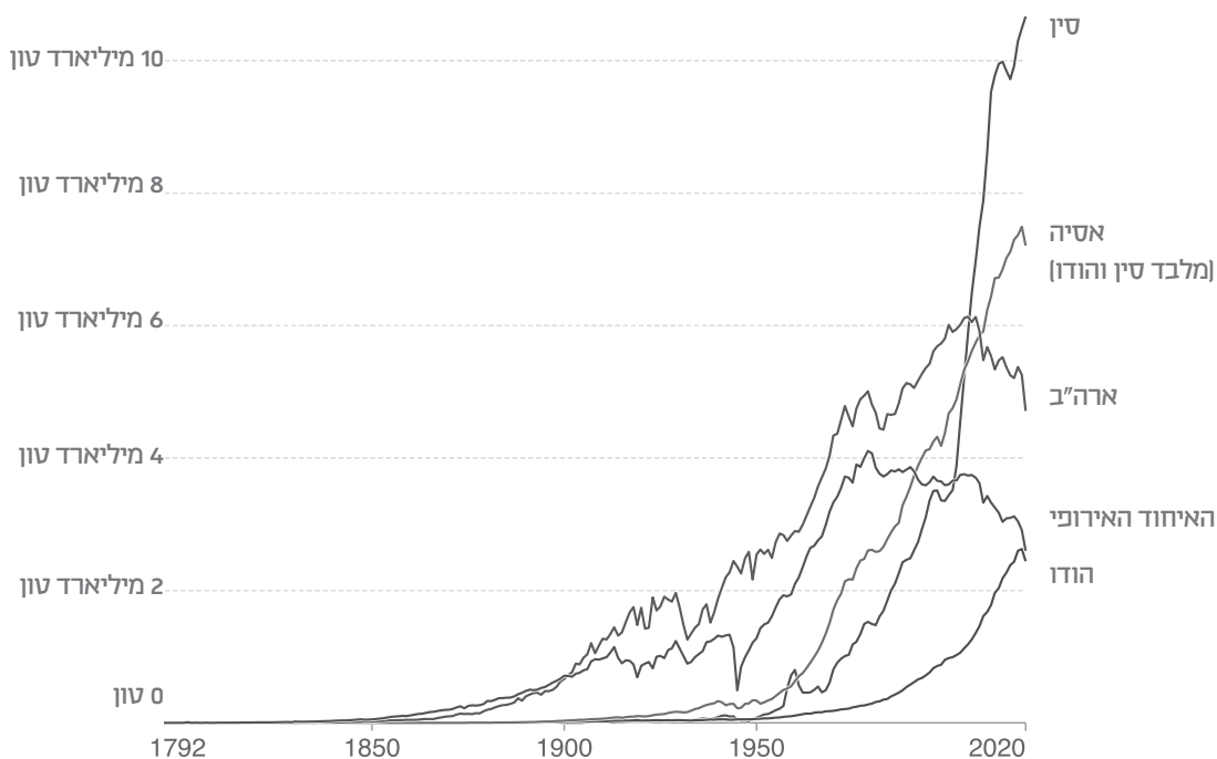
מקור הנתונים: Our World in Data / התרשים על פי Global Carbon Project
